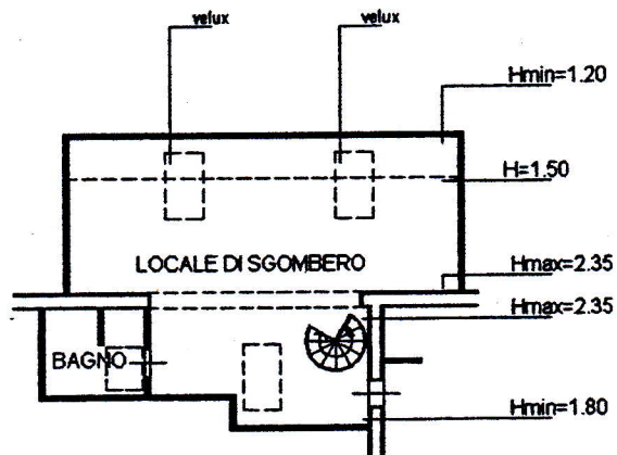
PIANO TERZO (SOTTOTETTO)
